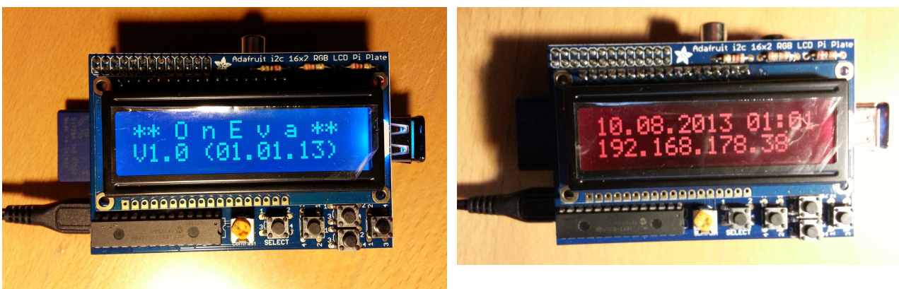
Abbildung 2: Komfortversion der Box
